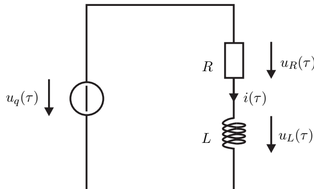
Abbildung 2: RL-Schwingkreis
